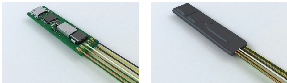
Рис. 1. CAN-реле
